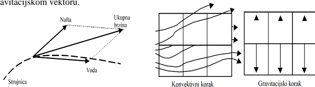
Slika 2-11. Ne poklapanje faznih vektora s vektorom ukupne brzine zbog utjecaja gravitacije (lijevo); Prikaz koraka rješavanja jednažbe materijalnog uravnoteženje nakon razdvajanja operatora (desno) (Thiele, 2005)
