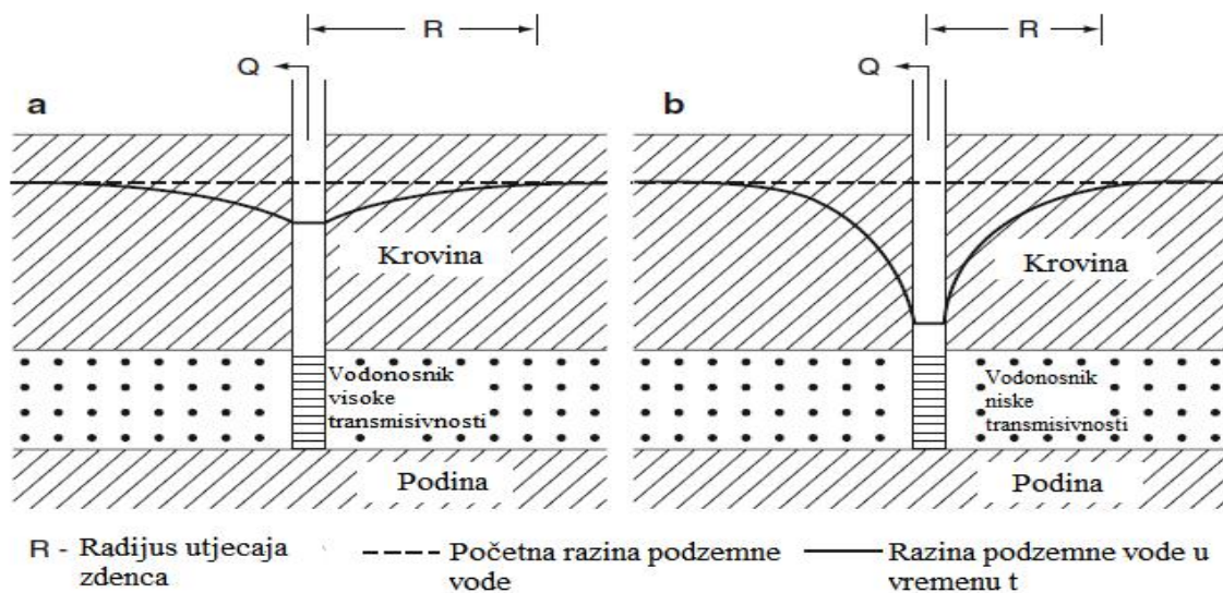
Slika 3.4. Prikaz sniženja vode nastalog uslijed crpljenja iz vodonosnika visoke (a) i niske (b) transmisivnosti
