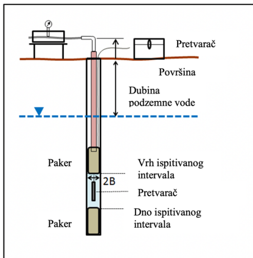
Slika 4.2. Mjerenje tlaka bušotinskim pretvaračem (Waterloo Hydrogeologic, 2020)
