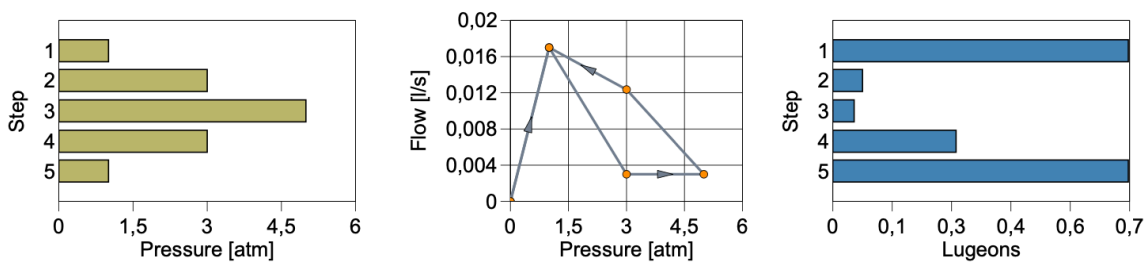
Slika 6.5. Dijagrami tlak-korak, tlak-protok i Lugeonova jedinica-korak za test broj 7
