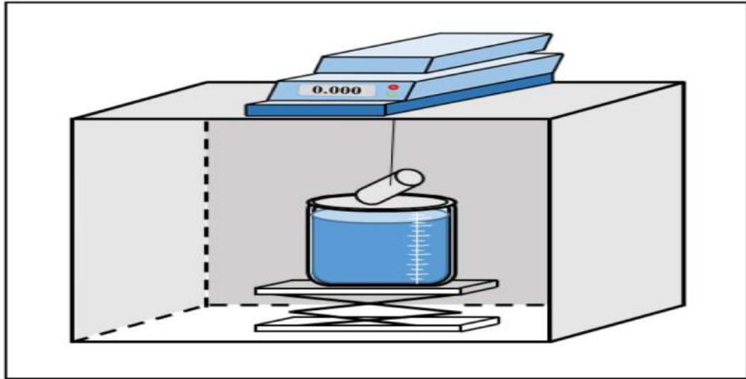
Slika 6-6. Prikaz uređaja pomoću kojeg se određivala masa izrezanih dijelova geopolimernog uzorka (Ahdaya et al., 2019)
