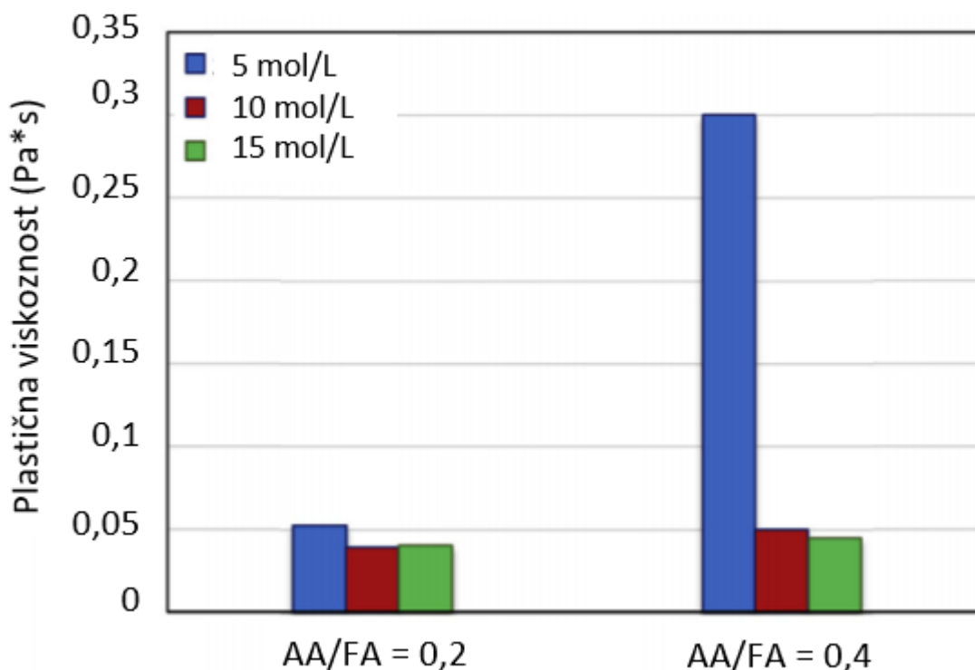
Slika 6-4. Utjecaj različitih AA/FA omjera i različitih koncentracija natrijevog hidroksida za SS/SH = 1 na plastičnu viskoznost geopolimernih cementnih kaša (Ahdaya et al., 2019)
