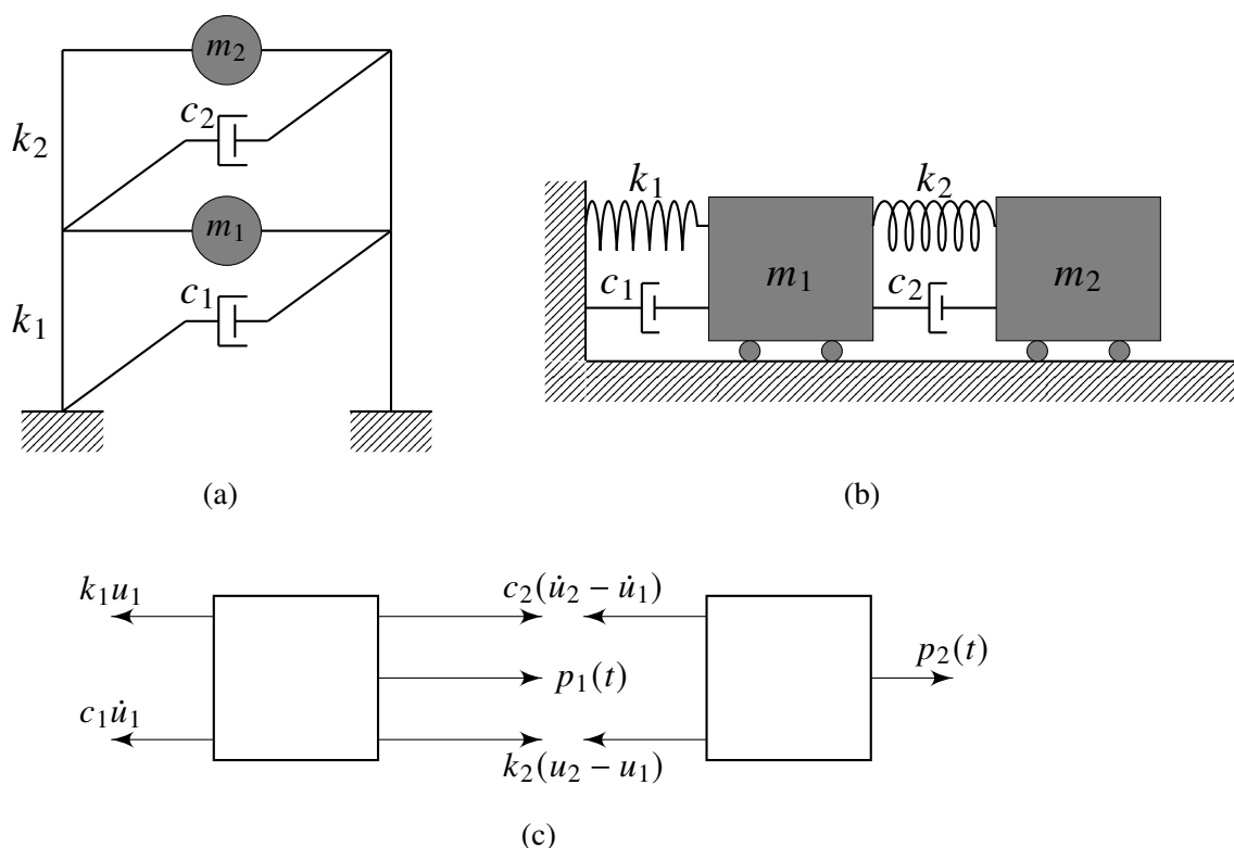
Slika 3.4: Idealizirani sustav s dva stupnja slobode i prigušenjem: (a) dvoetažni posmični okvir s prigušenjem; (b) ekvivalentni prigušeni model; (c) prikaz sila;
