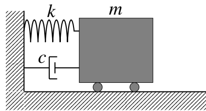
(b) Ekvivalentni model s prigušenjem
