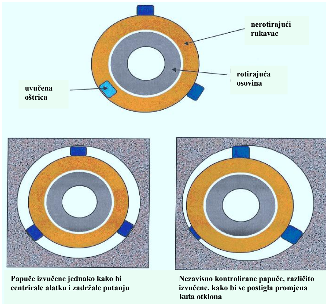
Slika 2-7. Hidrauličke papučice pri pravocrtnom i usmjerenom bušenju (Moody et al., 2004)
