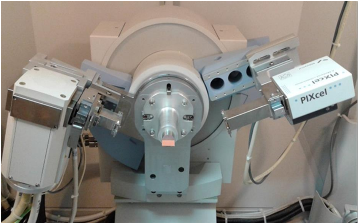
Slika 4-18. Rendgenski difraktometar Hrvatskog geološkog instituta
