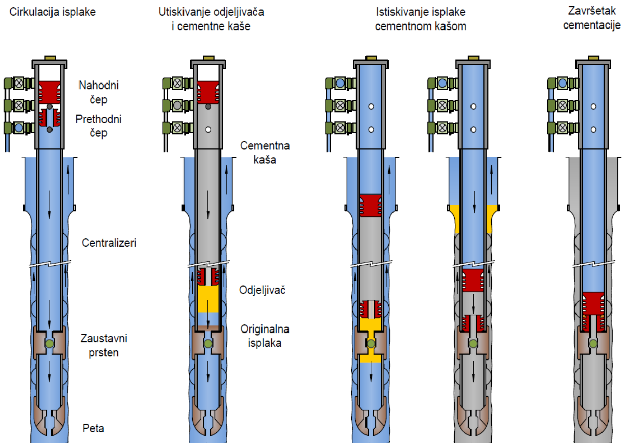
Slika 4-2. Shematski prikaz jednodimenzionalne cementacije kolone zaštitnih cijevi (Gaurina-Međimurec, 2017)
