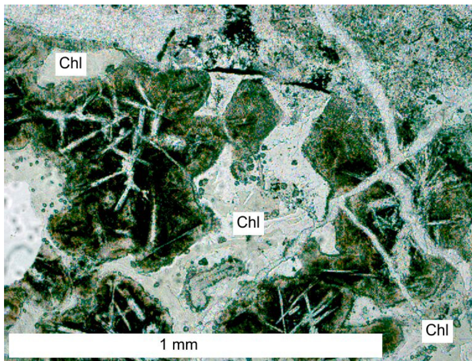
Slika 5-25. Sferuliti nastali procesom devitrifikacije u kojima su vidljivi mikroliti plagioklasa između kojih je vulkansko staklo alterirano u palagonit, a sve se nalazi u vulkanskom staklu devitificiranom u klorit (Chl) (Garašić, 2015)
