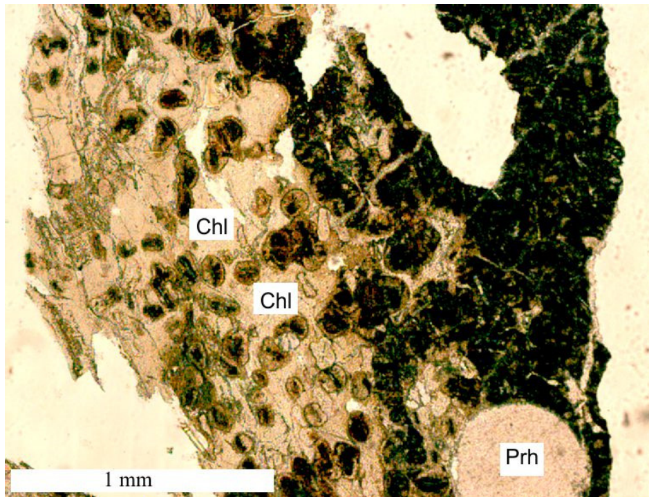
Slika 5-24. Dio vulkanskog stakla je devitificiran u klorit (Chl), sa sporadično razvijenim žuto-smeđim sferulitima, u kojima se kao i na krajnjem desnom dijelu fotografije razvija palagonit. Na slici je vidljiva i pravilna okrugla vezikula ispunjena prehnitom (Prh) (Garašić, 2015)
