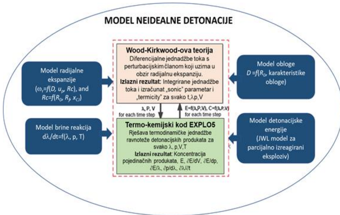
Slika 65. Elementi modela neidealne detonacije
