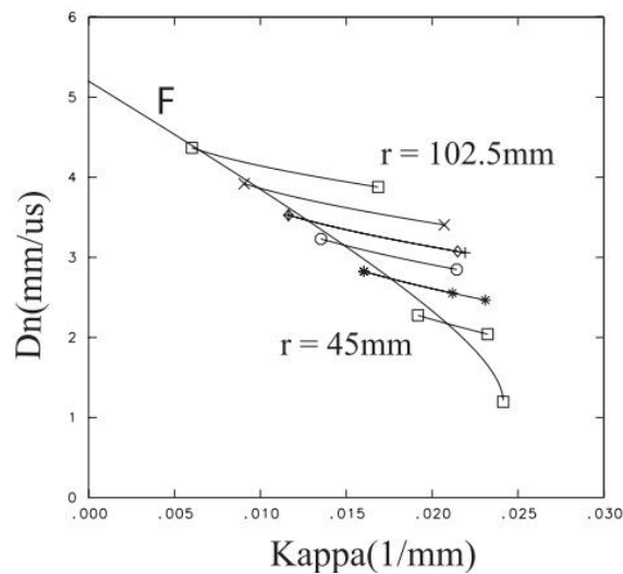
Slika 27. Primjer eksperimentalno dobivene ovisnosti brzine detonacije o zakrivljenosti kod ANFO eksploziva različitog radijuse naboja (Bdzil i ostali, 2002)
