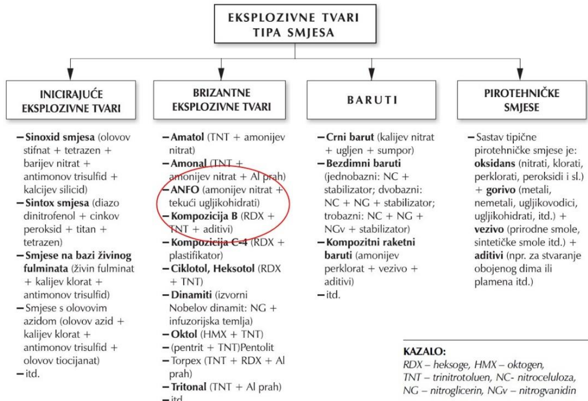
Slika 2. Podjela eksplozivnih smjesa (Sućeska, 2001)
