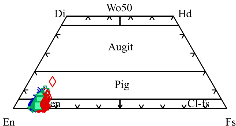
Slika 5.99. Klasifikacijski dijagram ortopiroksena (Morimoto, 1988) u ultramafitima Banovine. Plava boja – spinelski lercoliti S-pojasa; svijetlo zelena boja – lercoliti J-pojasa; tamno zelena boja – duniti J-pojasa; crvena boja – pirokseniti J-pojasa.
