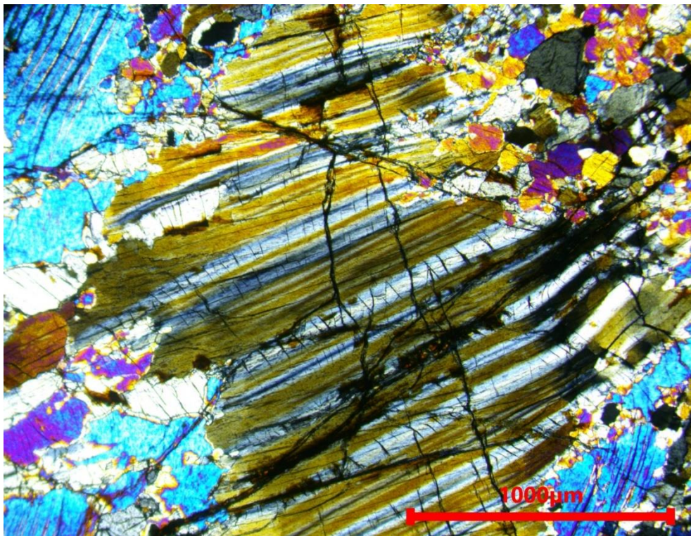
Slika 5.75. Vrlo široke eksolucijske lamelle ortopiroksena u klinopiroksenu vebsterita 18Gv-14, (N+).
