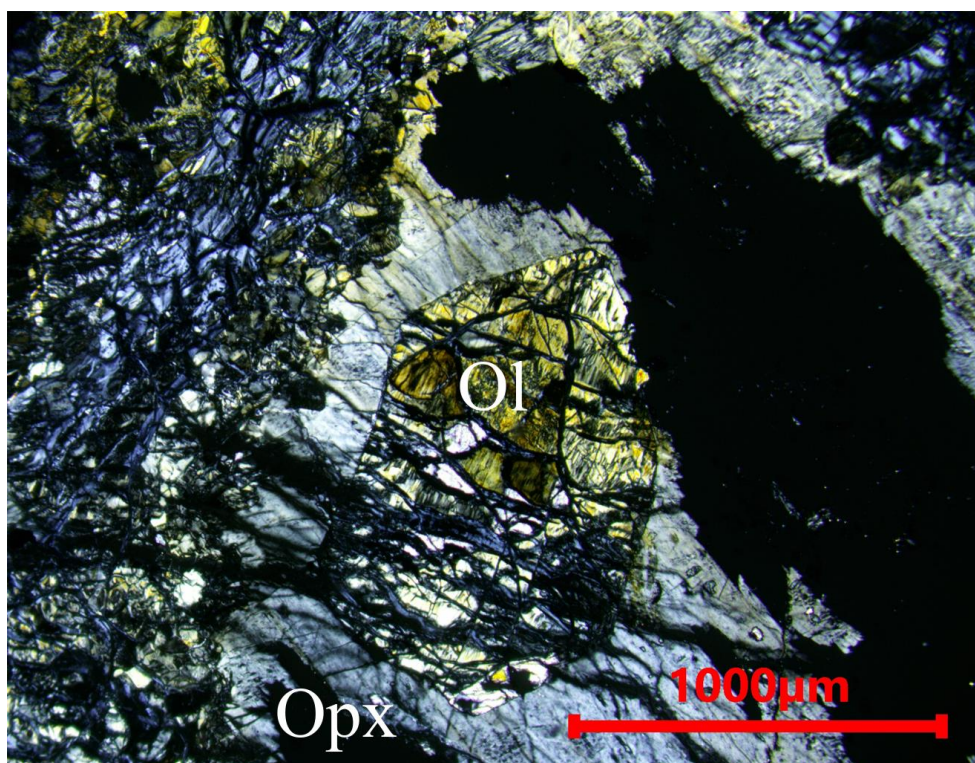
Slika 5.26. Inkluzija serpentiniziranog olivina u serpentiniziranom ortopiroksenu. Uzorak spinetskog lercolita LJ-3. Opx – ortopiroksen, Ol – olivin, (N+).
