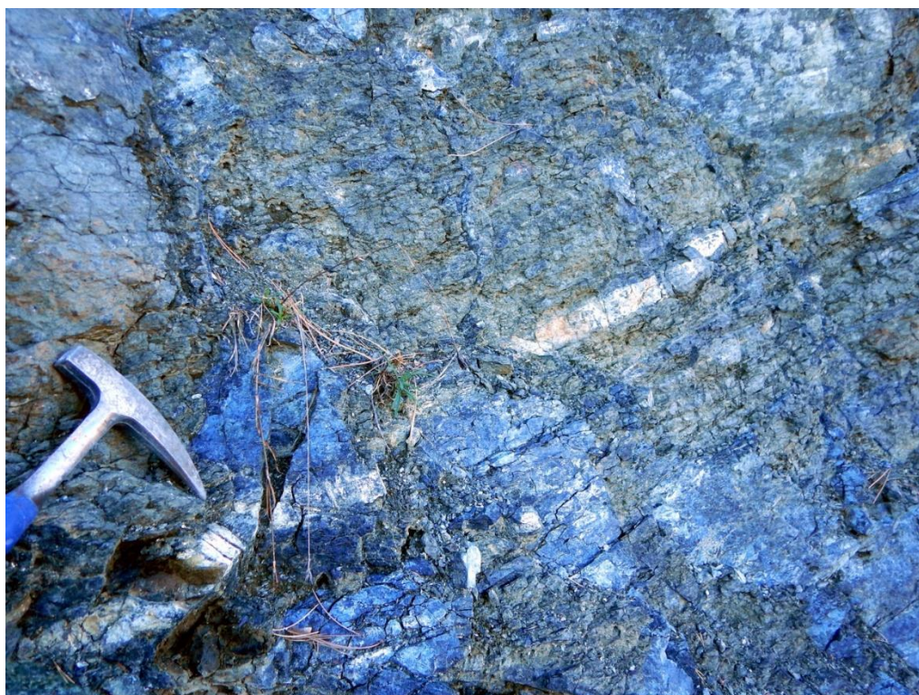
Slika 5.13 c. Trakaste forme, izmjena vebsterita (svijetla boja) i olivinskog vebsterita (tamna boja). Lokalitet Gvozdansko.
