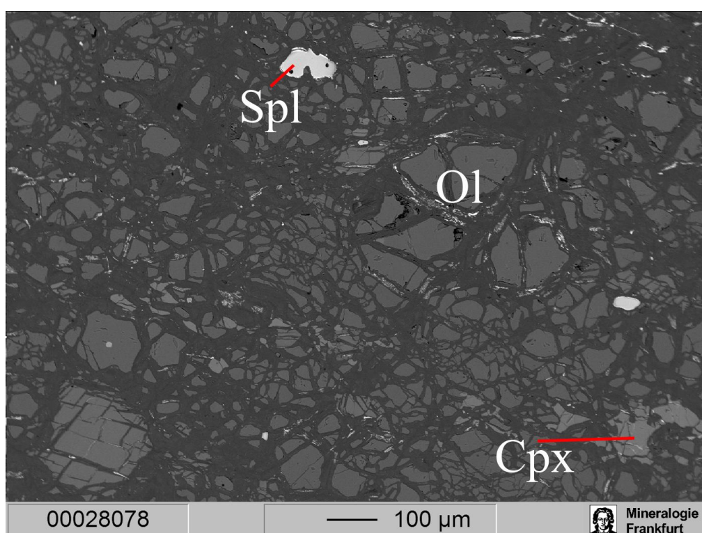
Slika 5.67. BSE snimka klinopiroksena u dunitu Gv-7. Ol – olivin, Cpx – klinopiroksen, Spl - spinel.
