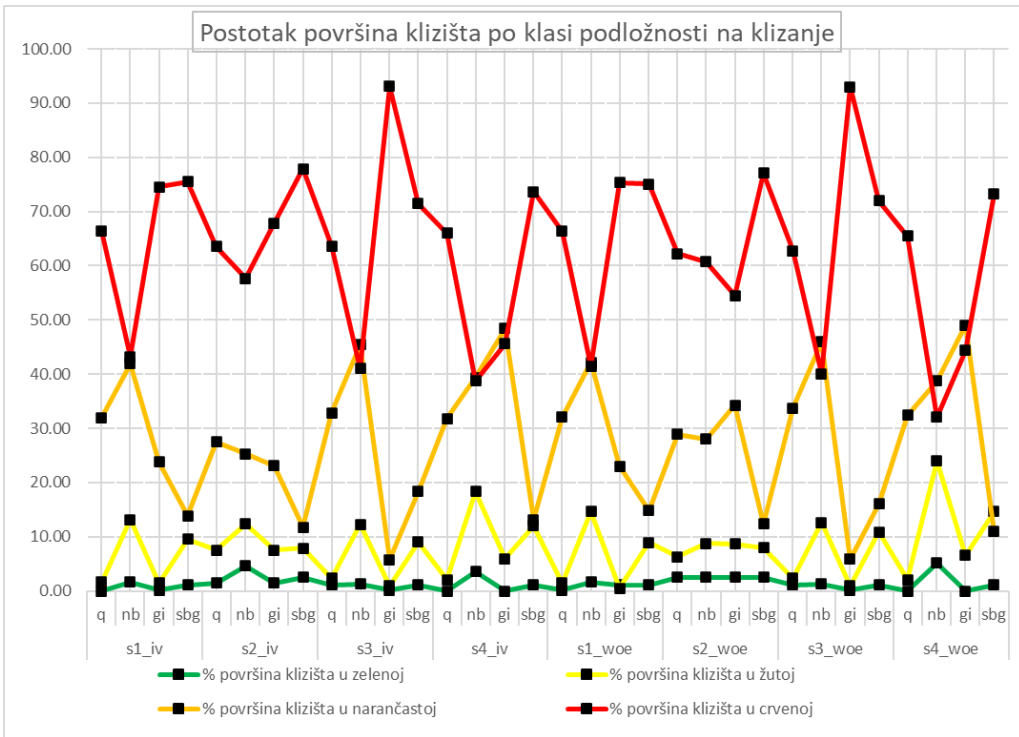
Slika 6.4 Udio površina klizišta po klasi podložnosti na klizanje za sve karte podložnosti
