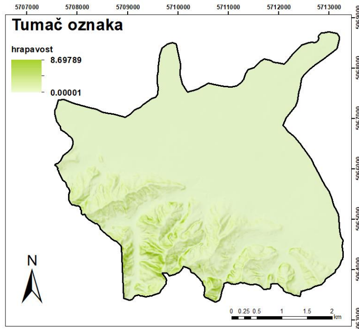
Slika 4.8 Hrapavost terena istraživanog područja
