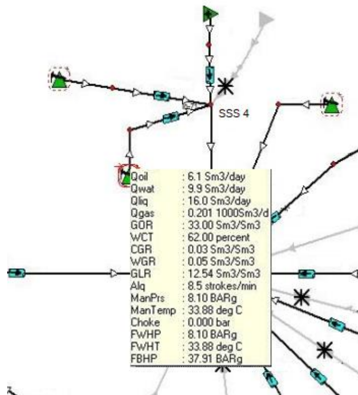
Slike 4-18. Dobiveni podaci za bušotinu X-1
