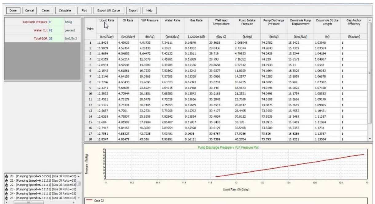
Slika 4-10. Prikaz proračuna i izгледа VLP krivulje
