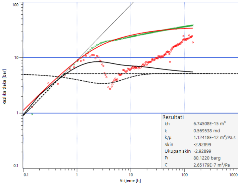
Slika 4-11. Log-log dijagram analize testa porasta tlaka – analiza 2
