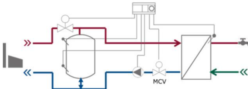
Slika 3-7. DHSU toplinska stanica (Schmidt et al., 2017)
