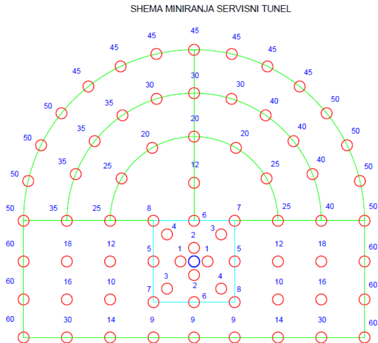
Slika 5.3-2 Shema miniranja za servisnu cijev tunela (OpusGEO, 2017.)
