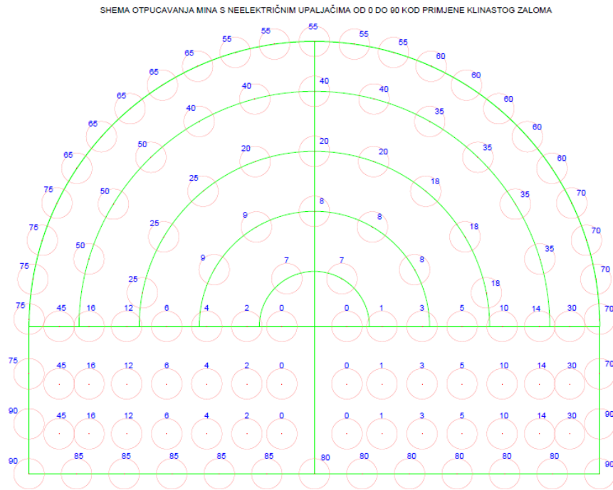
Slika 5.3-1 Shema miniranja za glavnu cijev tunela (OpusGEO, 2017.)
