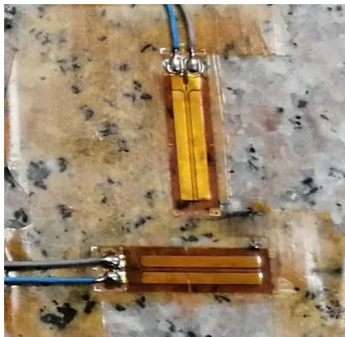
Slika 3-14. Zalijepljene mjerne trake.
