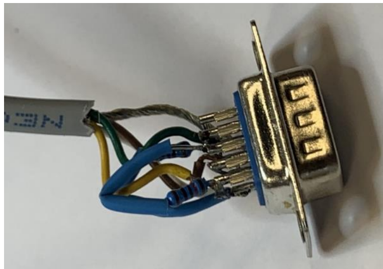
Slika 3-12. Zalemljeni konektor.
