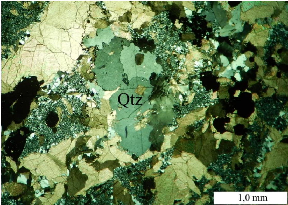
Slika 2-3. Polikristalno zrno kvarca (+N).
