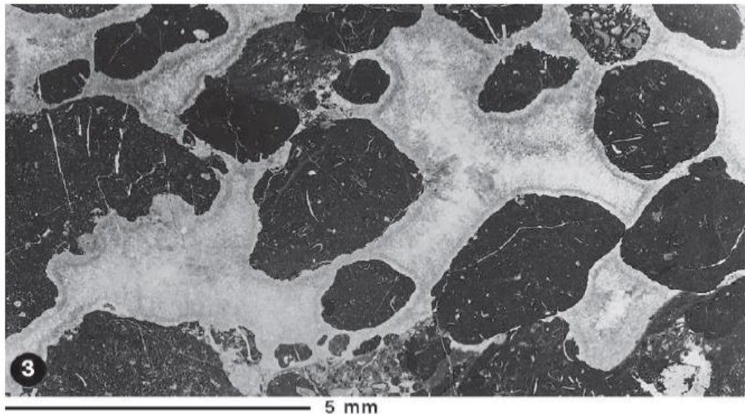
Slika 3 Monomiktne karbonatne breče sa međuzrnskom potporom; preuzeto iz Flügel (2004)
