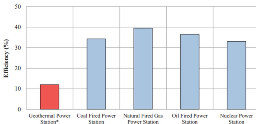
Slika 3 Učinkovitost geotermalne elektrane u usporedbi s ostalim termoelektranama (Zarrouk & Moon 2013)
