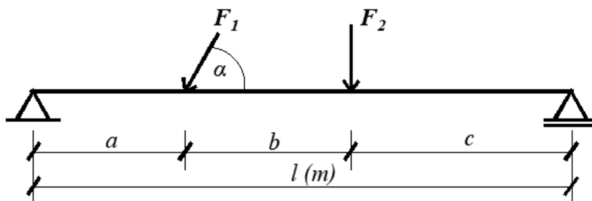
Slika 4-1 Jednostavna greda
