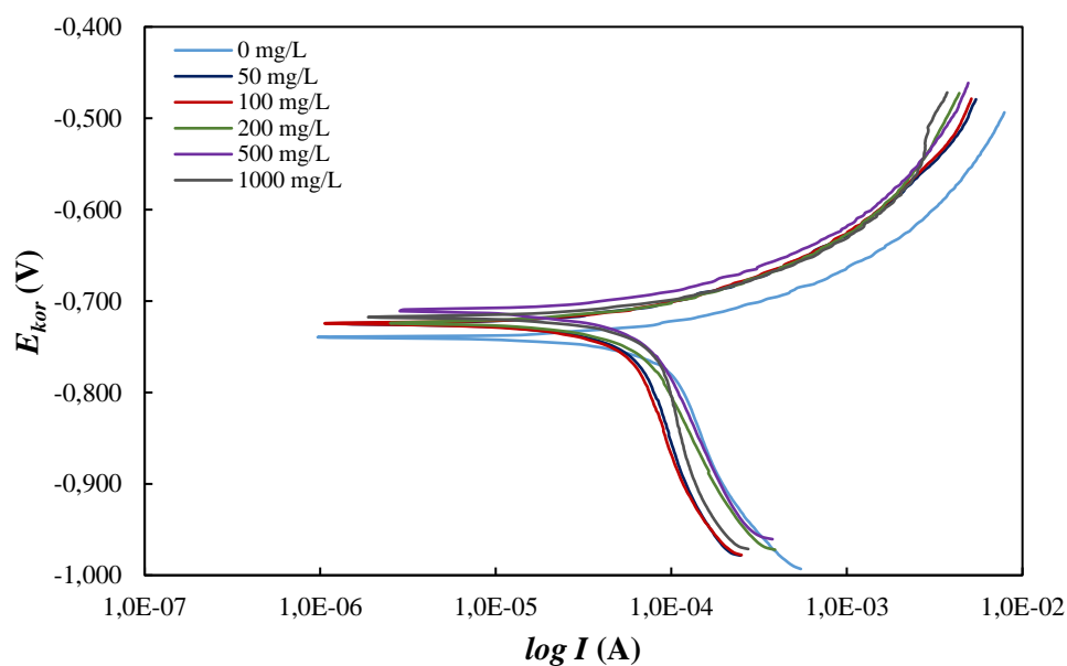
Slika 5-3. Polarizacijske krivulje snimljene na uzorku ugljičnog čelika u simuliranoj slojnoj vodi zasićenoj s \text{CO}_2 za različite koncentracije ekstrakta matičnjaka
