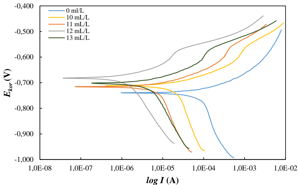
Slika 5-35. Polarizacijske krivulje snimljene na uzorku ugljičnog čelika u simuliranoj slojnoj vodi zasićenoj s CO 2 bez i u prisutnosti različitih koncentracija ekstrakta korijena maslačka
