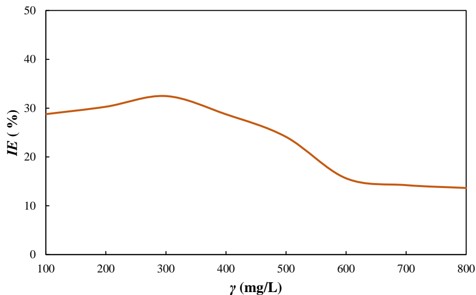
Slika 5-8. Inhibitorska djelotvornost ekstrakta pasiflore u ovisnosti o koncentraciji
