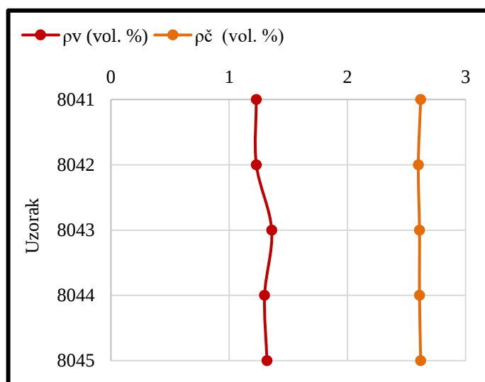
Slika 4.10. Grafički prikaz distribucije volumnne gustoće ( \rho_v ) i gustoće čvrstih čestica ( \rho_{\check{c}} ) na profilu Terra Rosse.
