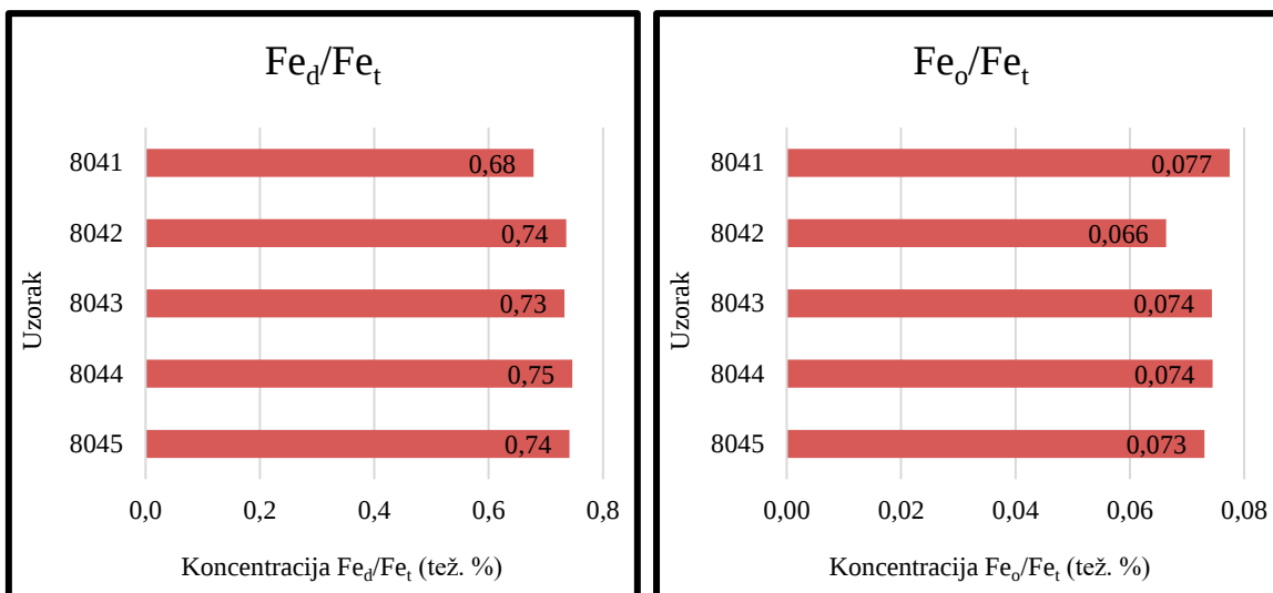
Slika 4.16. Dijagrami udjela omjera ditionit topivog željeza (Fe d ) i ukupnog željeza (Fe t ) (lijevo) i omjera oksalat topivog željeza (Fe o ) i ukupnog željeza (Fe t ) (desno) u uzorcima Terra Rosse.
