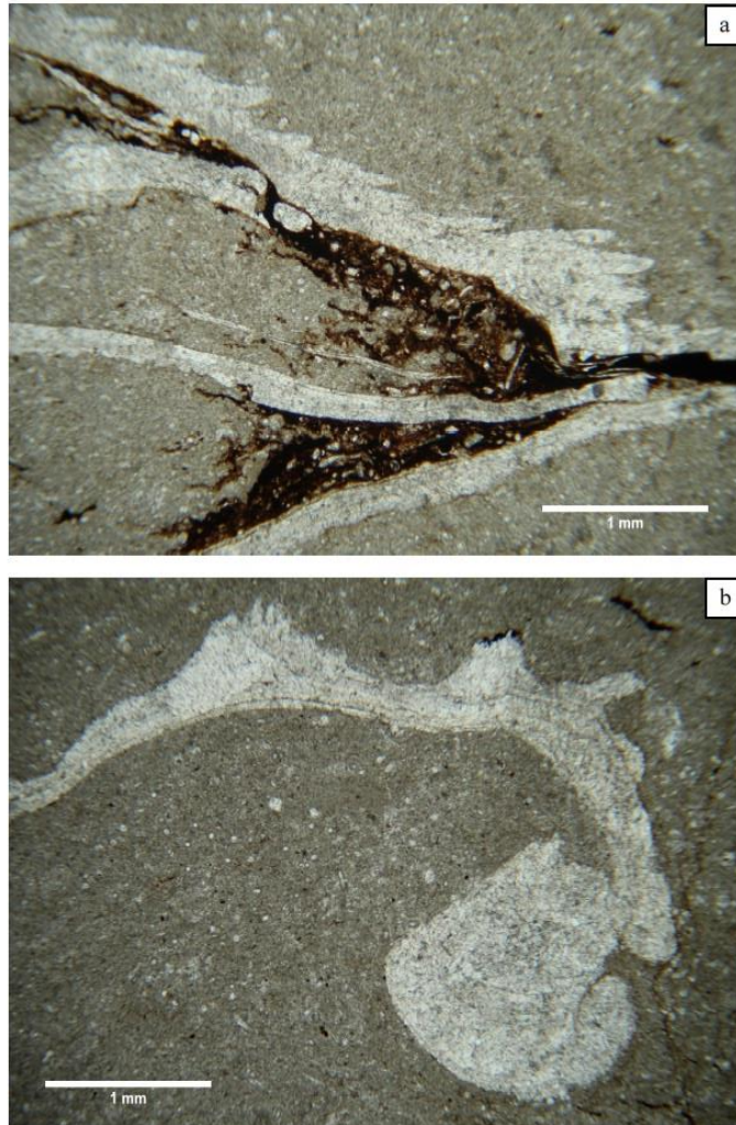
Slika 8 - 9 Mikrofotografije uzorka vapnenca M-11: a) rub ljuštine školjkaša; b) fragment gastropoda.
