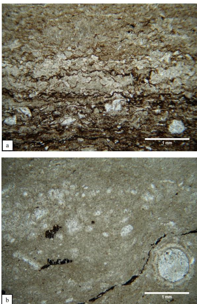
Slika 8 - 6 Mikrofotografije uzorka vapnenca M-3: a) jasno vidljiva laminacija; b) u donjem desnom kutu vidljiva je zelena alga.
