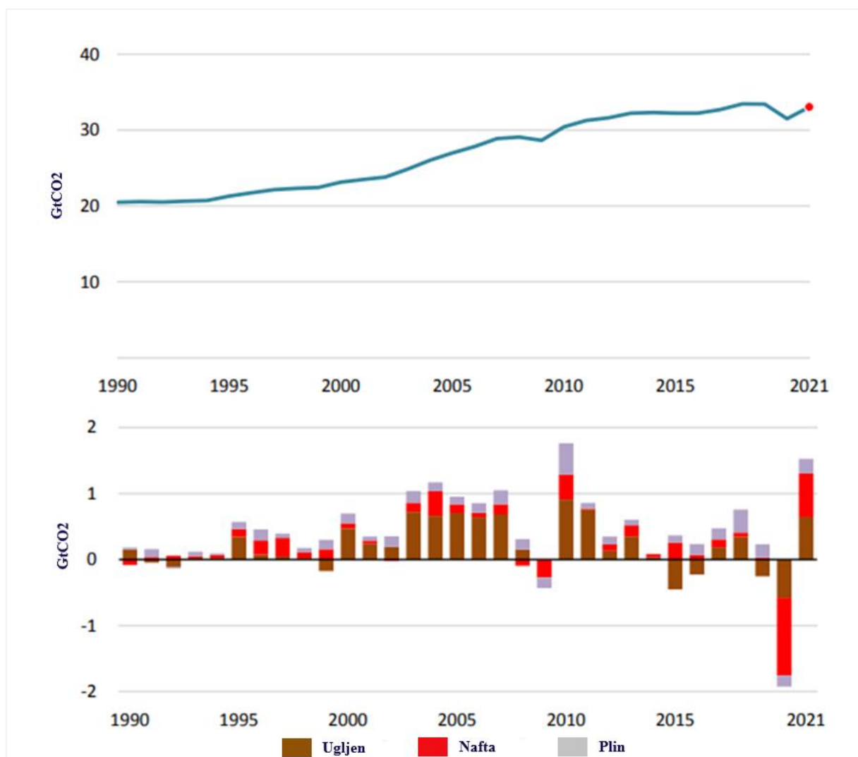
Slika 5-2. Globalne emisije CO 2 iz primarne energije i promjena u emisijama CO 2 prema gorivu, 1990. – 2021. (prema IEA, 2021a)
