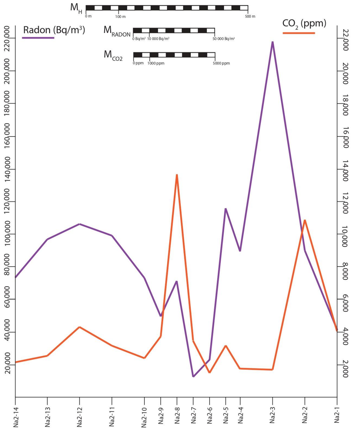
Slika 24. Izmjerene koncentracije radona i CO 2
