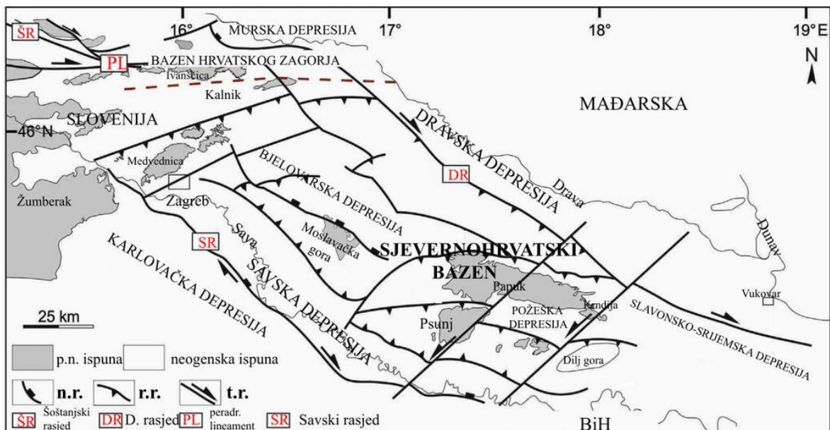
Slika 4. Karta prikaza rasjeda, podloge neogena i neogenske ispuna na području Sjevernohrvatskog bazena ( Pavelić i Kovačić, 2018 )
