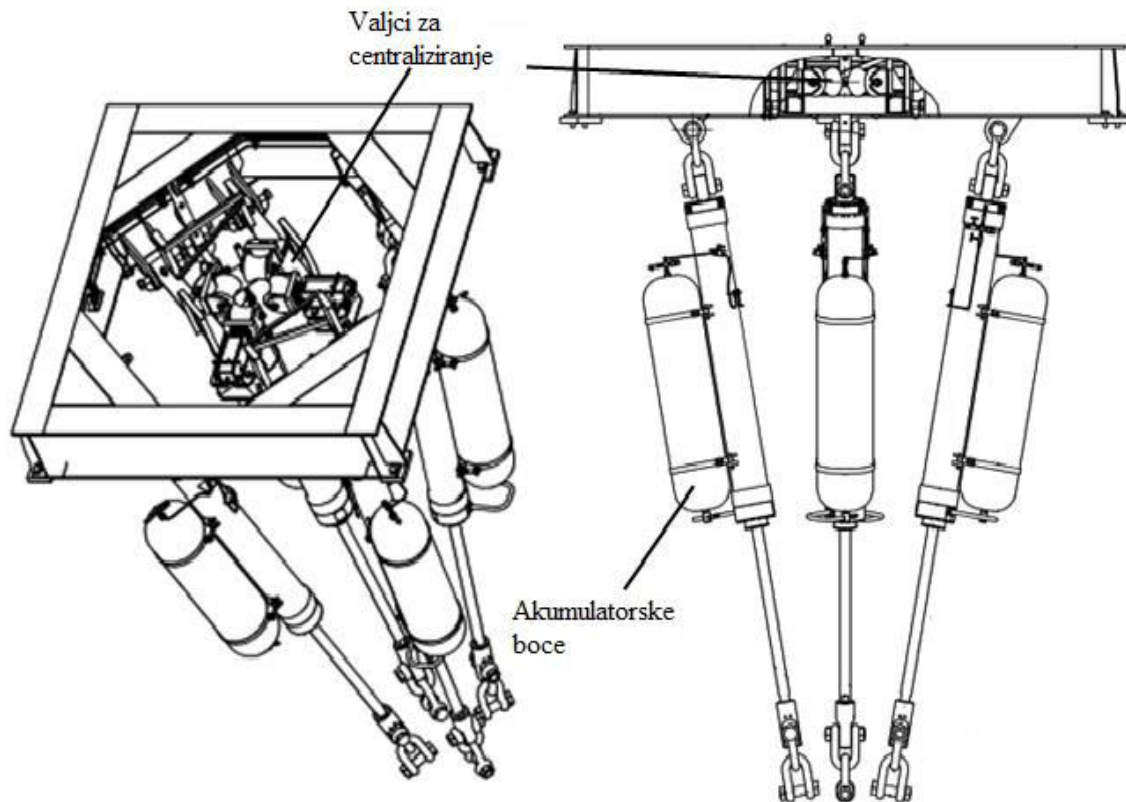
Slika 2-14. Kizomba TLP proizvodni natezni sustav (Dunn 2013)
