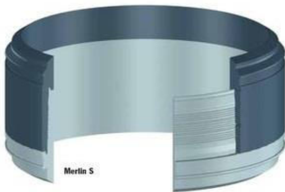
Slika 3-6. Merlin spojnice (www.oilstates.com)
