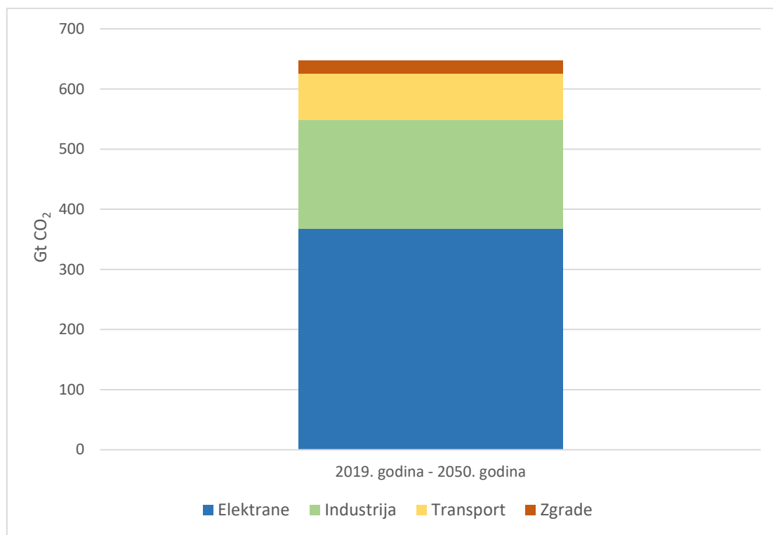
Slika 2-3. Emisije CO 2 u svjetskom energetskom sektoru iz postojećih energetskih i industrijskih postrojenja, 2019. godine - 2050. godine (prema IEA, 2020)
