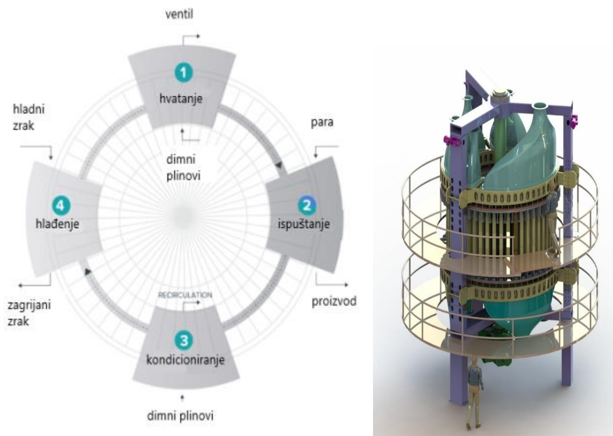
Slika 5-2. Inventys' VeloxoTherm TM procesa koji je osmislila kompanija Svante (prema Svante, BCTechnology, 2017)
