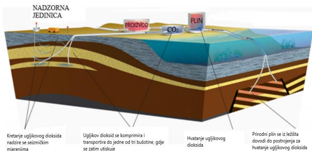
Slika 4-3. CCS projekt Gorgon u Australiji (prema Chevron, 2019)
