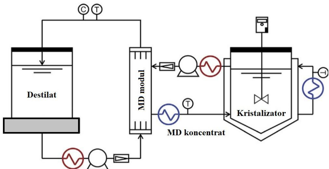
Slika 5-5. Shema MDC procesa (Li et al., 2019)
