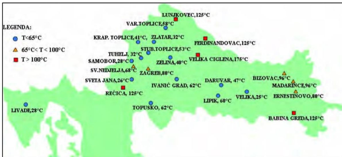
Slika 7-2. Geotermalni resursi Hrvatske (Dekanić et al., 2008)
