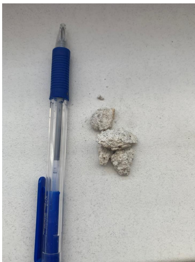
Slika 5.4. Fotografije uzorka MT61
