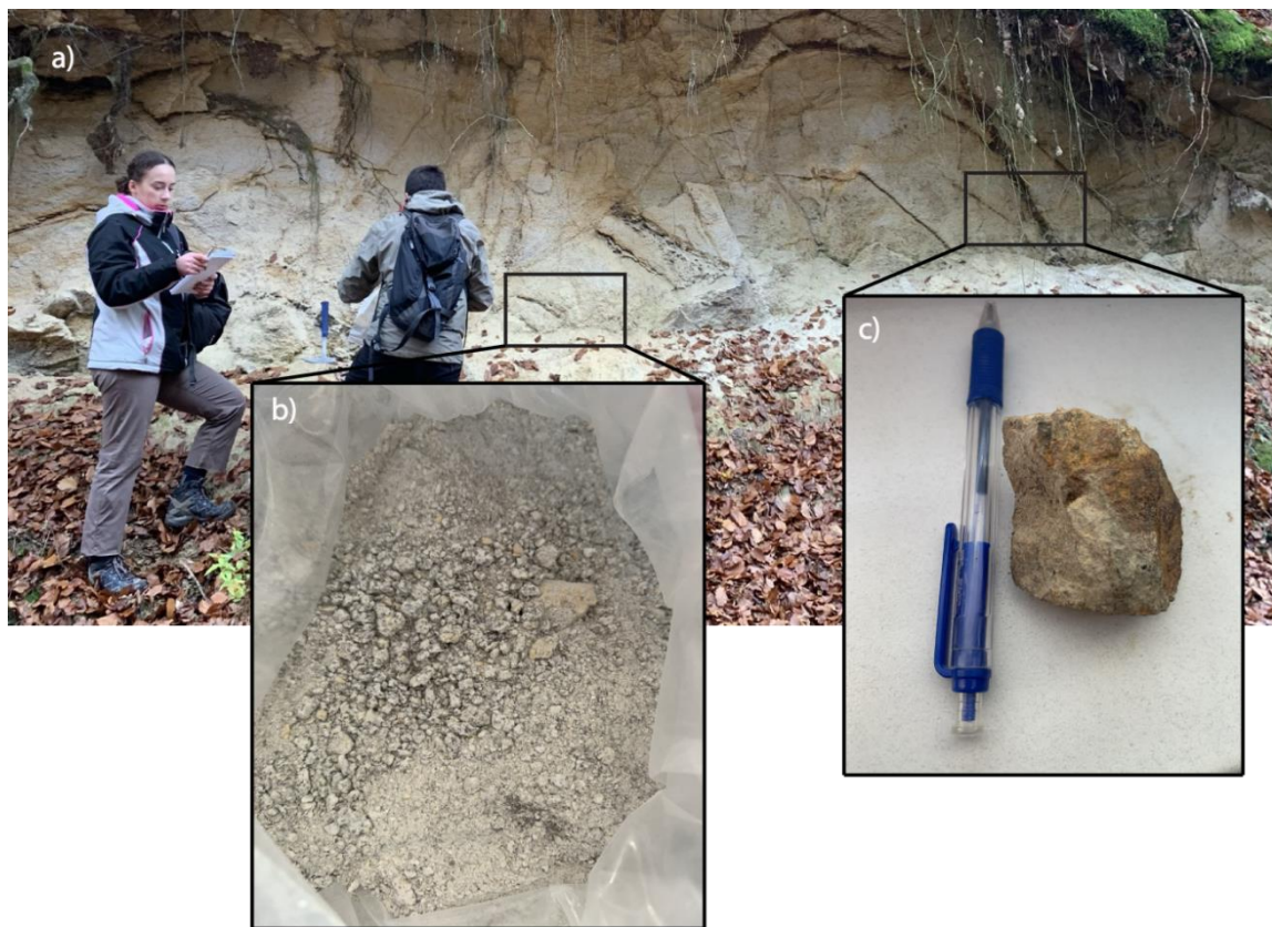
Slika 5.8. a) Snimak terena s označenim lokacijama uzorkovanja b) Fotografija uzorka MT68 c) Fotografija uzorka MT67
