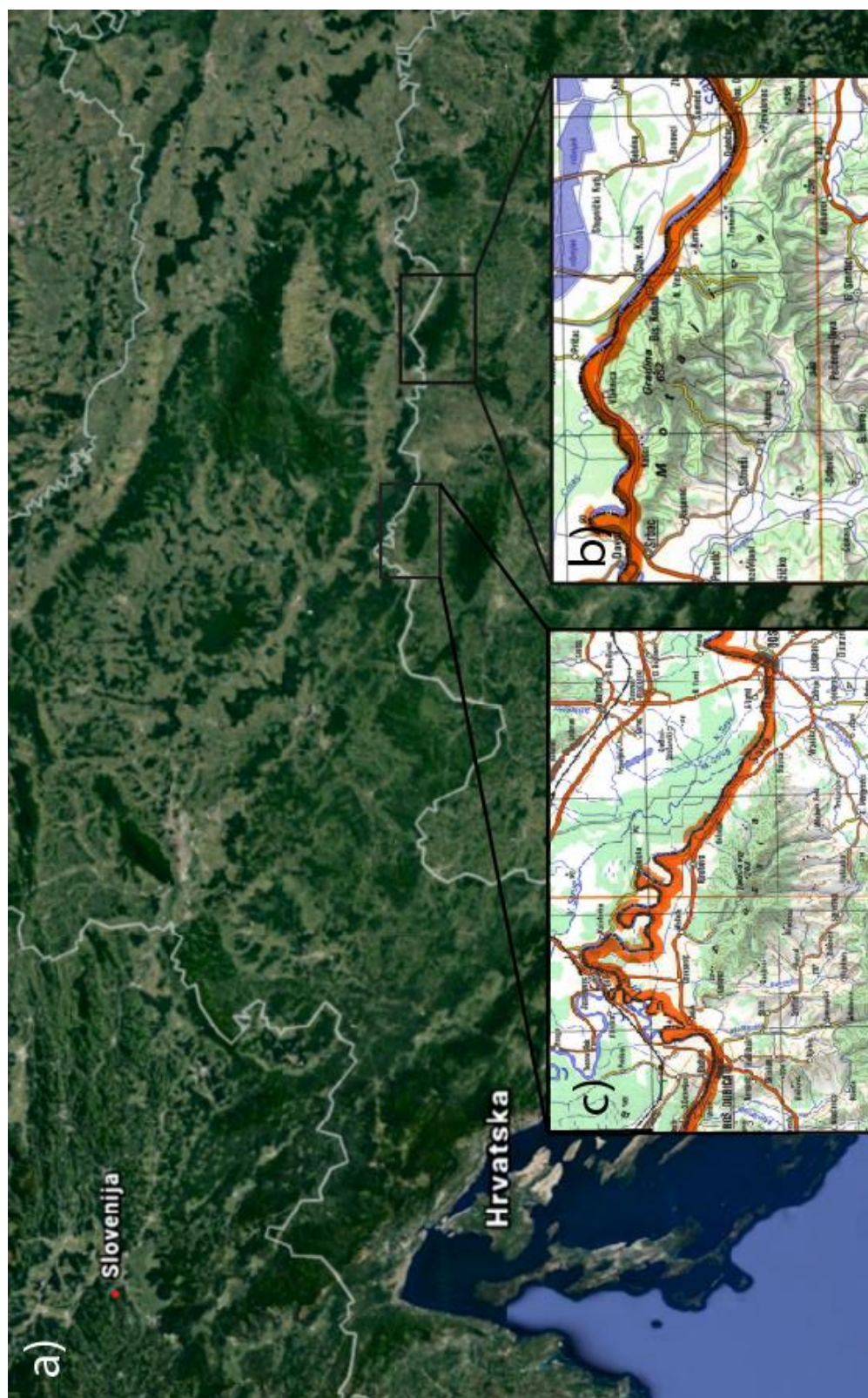
Slika 2.1. Geografski položaj istraživnog terena u odnosu na susjedne države. b) Isječak topografske karte Motajice izvornog mjerila 1 : 300 000 (Dinarsko gorje: Motajica. URL3). c) Isječak topografske karte Prosare izvornog mjerila 1 : 300 000 (Dinarsko gorje: Prosara. URL4)
