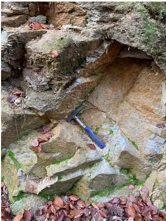
Slika 5.5. Fotografije uzorka MT62
