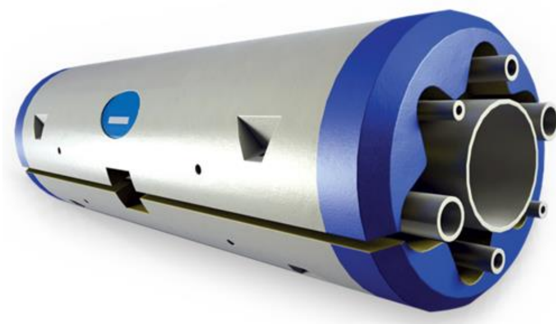
Slika 3-5. Prikaz usponske cijevi obložene uzgonskim modulom (www.crpsubsea.com, 2022)
