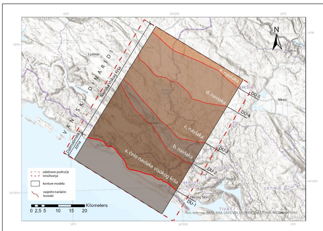
Slika 5.3 Površinska distribucija navlačnih ploha rasjeda u ArcGis Pro softveru. Na slici su vidljivi rasjedni poligoni s označenim presječnicima vršnih i baznih dijelova svake rasjedne plohe zasebno (a–e).
