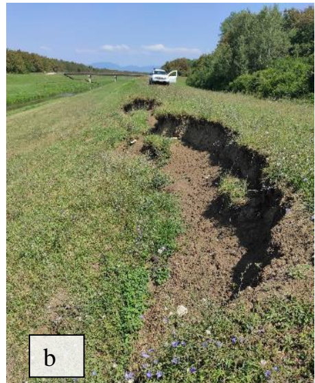
Slika 6.4 Klizište na nasipu: (a) trenutno neaktivno rotacijsko klizište; (b) recentno klizište s vidljivom glavnom pukotinom
