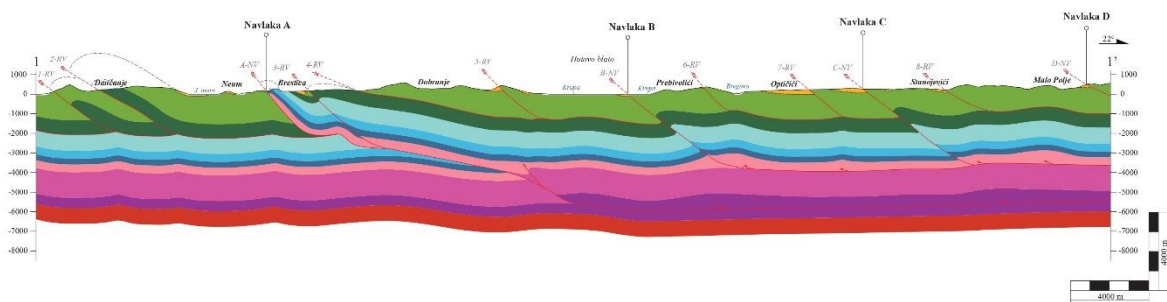
Slika 6.3 Geološki profil 1–1'.
