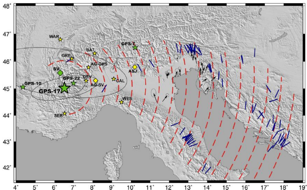
Slika 4.3 Prikaz lokacija izvedenog Eulerovog pola rotacije prema Weber et al. (2010) (zeleno – GPS-7, GPS-10, GPS-17, GPS-22, i SV (slip vector) koji odgovara GPS rješenjima za 7, 10, 17 i 22 mjesta), uspoređenih s prethodno objavljenim rješenjima (žuto): A&J – Anderson & Jackson (1987); WES – Westaway (1992); RAT – Ward (1994); CAL – Calais et al. (2002); BAT – Battaglia et al. (2004); GRE – Grenerczy et al. (2005); SER – Serpelloni et al. (2005); DEV – Devoti et al. (2008); AG-GPS – D'Agostino et al. (2008). Trajektorije i orijentacija vektora pomaka prikazani su crvenim i plavim crtama (Weber et al., 2010).
