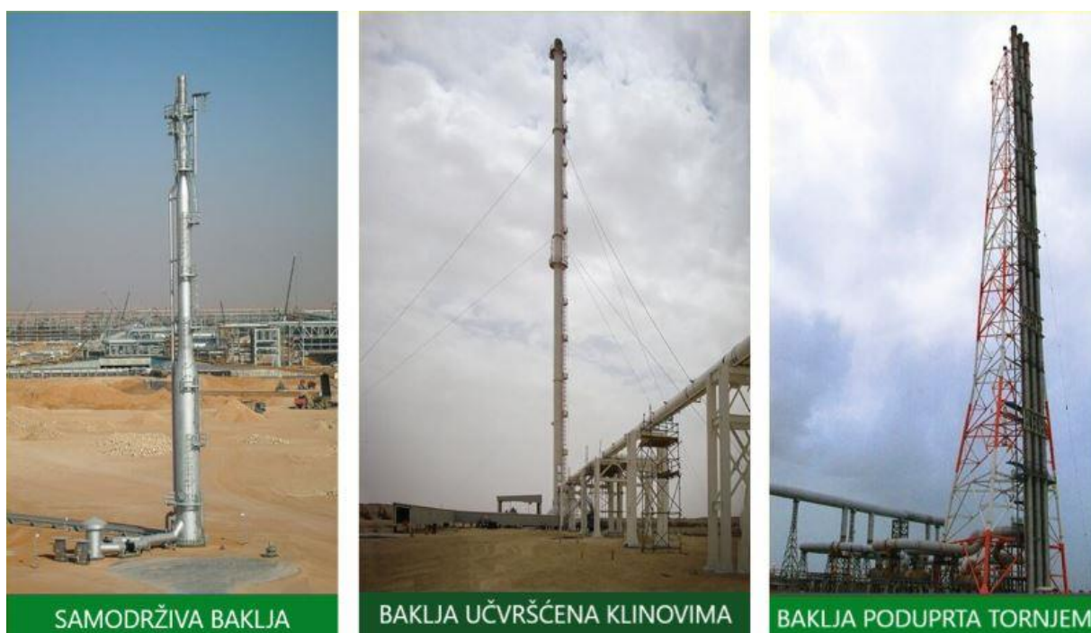
Slika 3-2. Tipovi konstrukcije uspravnih baklji (The piping talk, 2021)
