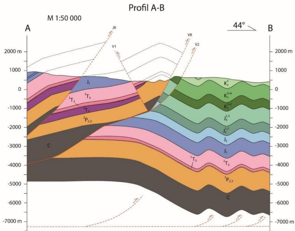
Slika 3-6. Interpretacija struktarno-geološke građe u području između Vrbovskog i Moravica prema Šegović (2020). Gore: položaj profila A-B na OGK list Črnomelj sa smjerom pružanja 44-224^\circ . Dolje: struktarno-geološki profil A-B koji prikazuje reversni rasjed s nagibom prema JZ i četiri glavna segmenta: rampe nagiba 63^\circ , zaravni s kutom nagiba 18^\circ , rampe nagiba 32^\circ i zaravni s kutom nagiba 20^\circ .
