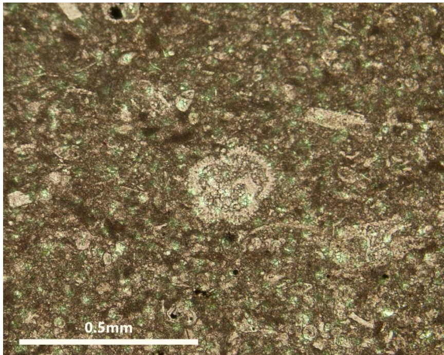
Slika 5-13. Globigerina (sredina fotografije) u uzorku TG13.
