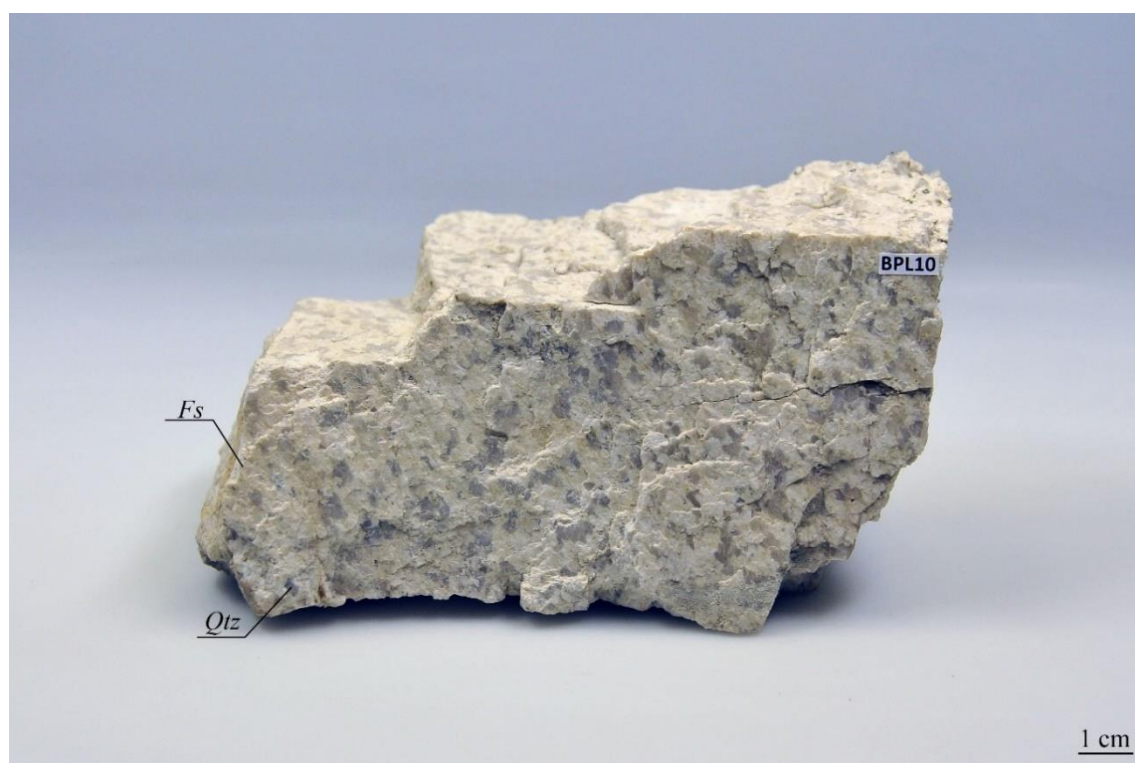
Slika 5-3 i: Alteracije u Cu-porfirnom ležištu (BPL10)
