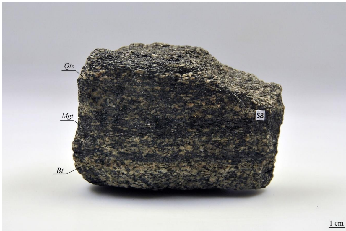
Slika 5-2 h: Željezoviti skarn (S8)
