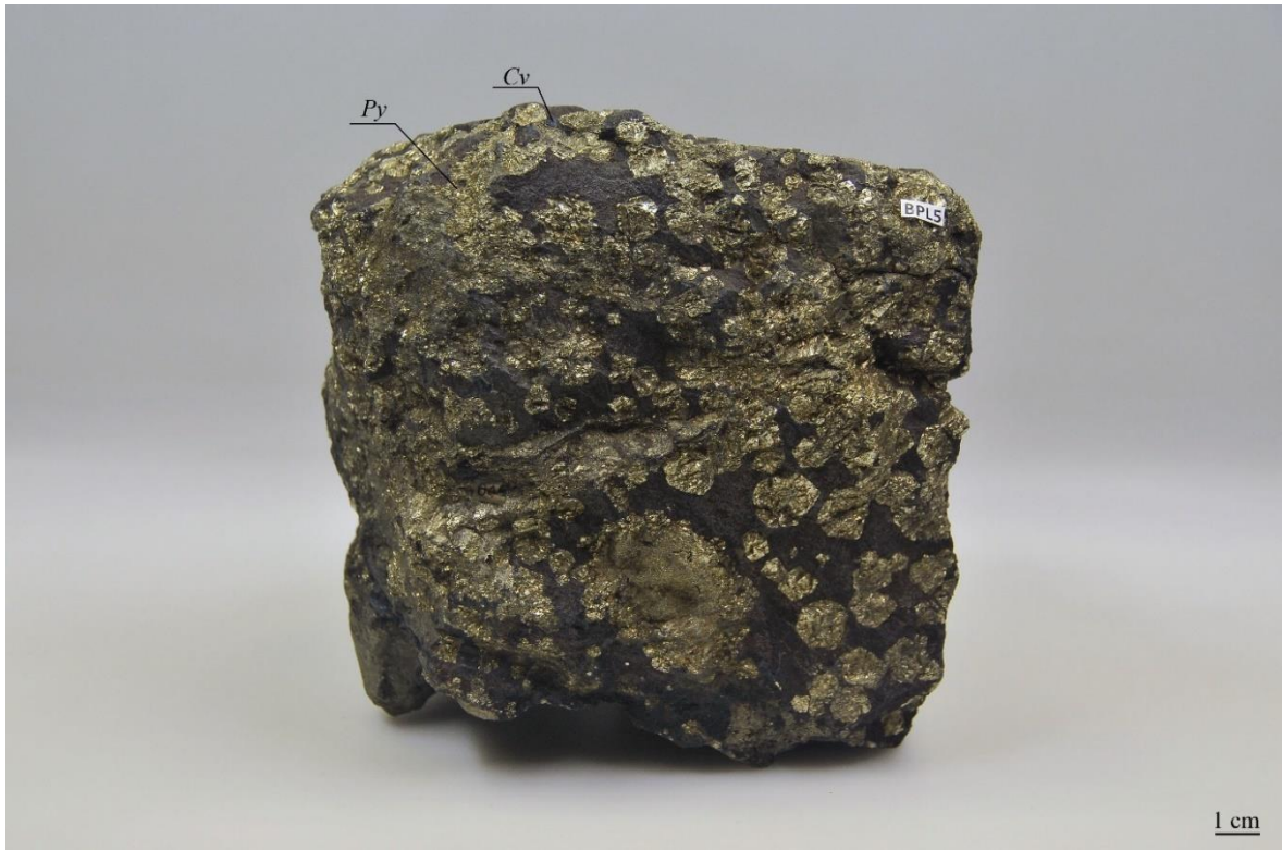
Slika 5-3 d: Cu-porfirna ruda (BPL5)
