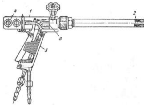
Slika 6-2. Termorezač model TR-14/22-5 (SSSR) (Dunda, 1989) 1-tijelo, 2-mlaznica, 3-komora izgaranja, 4-glava, 5-rukohvat
