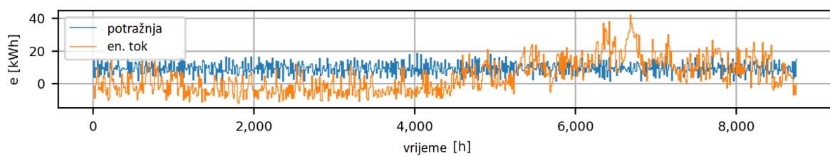
Slika 3-19. Potražnja električne energije i tok električne energije na godišnjoj razini – Broj bušotina +20%
