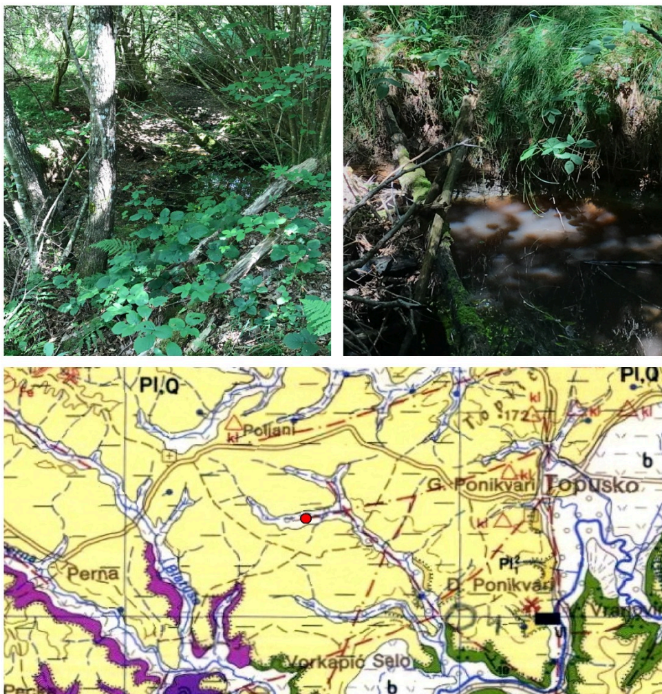
Slika 4-45. Lokacija pojave točke prijelomnice za sliv Crna Rijeka (lokacija, \varphi -45.2908342704599, \lambda -15.929864309743)
