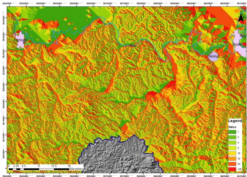
Slika 4-12. Smjer otjecanja površinskih tokova (engl. Flow Direction)
