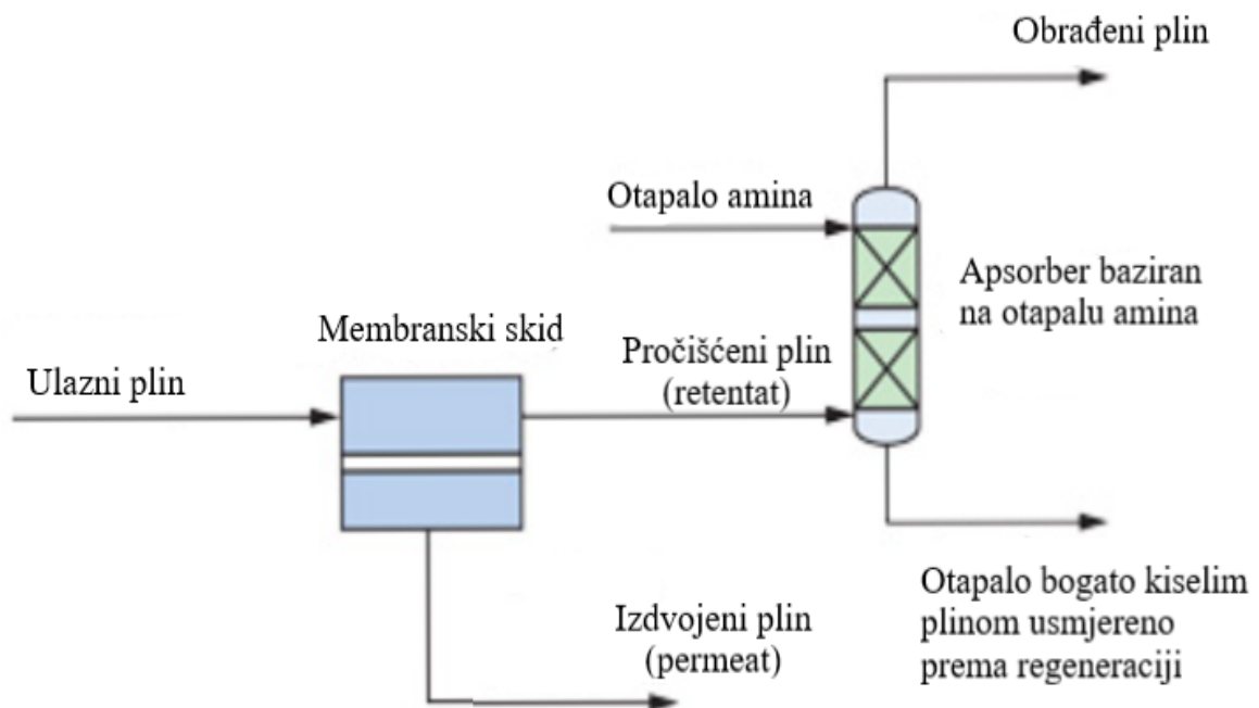
Slika 6-1. Hibridni proces membrane i kemijske apsorpcije aminima (Gas processing & LNG, 2022)
