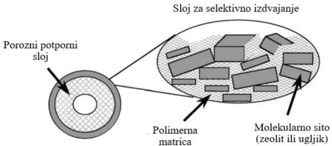
Slika 5-7. Shema mješovite matrične membrane (Shekhawat et al., 2003)
