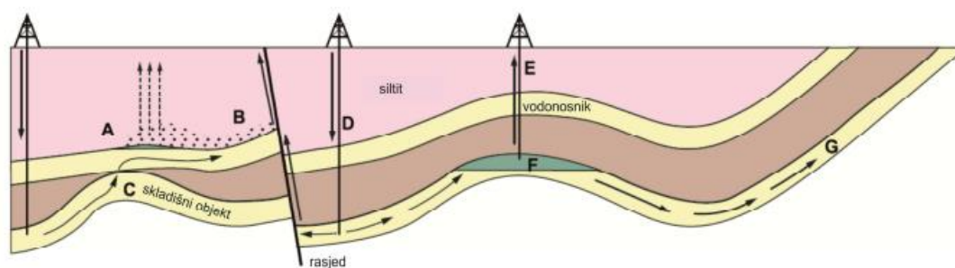
Slika 4-2: Potencijalni putevi migracije utisnutog CO 2 u pliće slojeve (IPCC, 2005)
