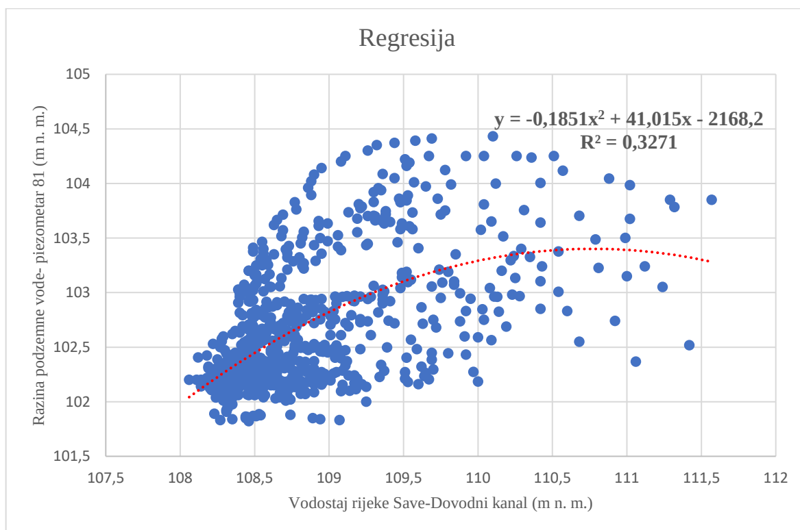
Slika 5.13: Prikaz rezultata polinomne regresije vodostaja Save Dovodni kanal TE-TO i piezometra 81 s jednadžbom polinoma II. Stupnja i koeficijentom determinacije
