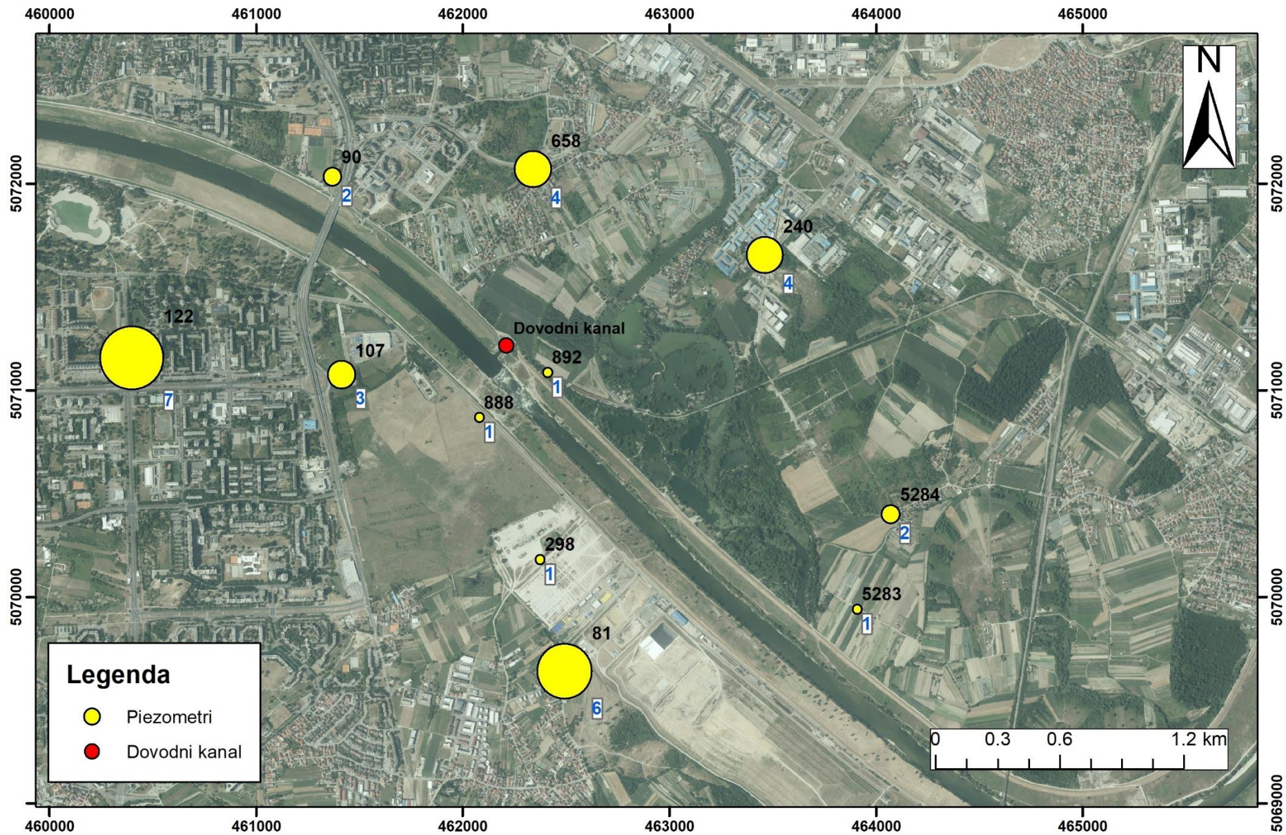
Slika 5.36: Prikaz piezometara sa vremennskim zaostajanjima (naziv piezometra označen je crnom bojom, a vremensko zaostajanje plavom bojom)
