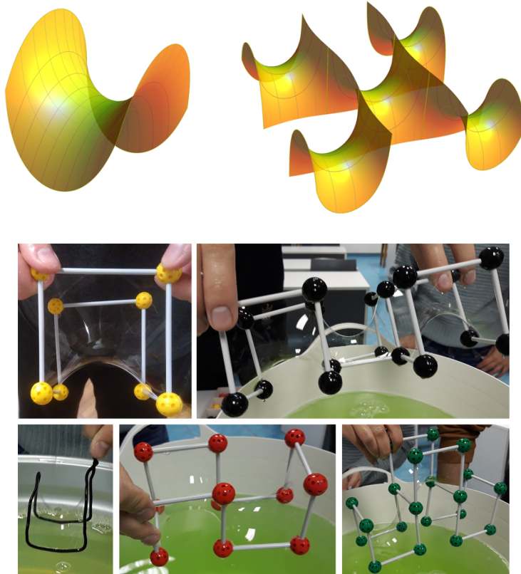
Slika 7. Scherkova ploha i njene generalizacije
