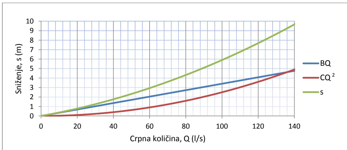
Slika 5-7. Dijagram s=f(Q) i pojedine vrste gubitaka za dvosatno crpljenje zdenca ZK-1
