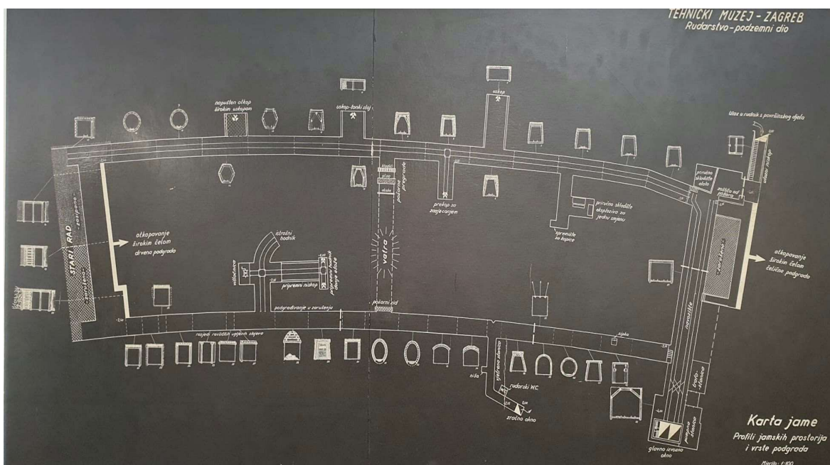
Slika 1-1. Tlocrt rudnika, Tehnički muzej Nikola Tesla
