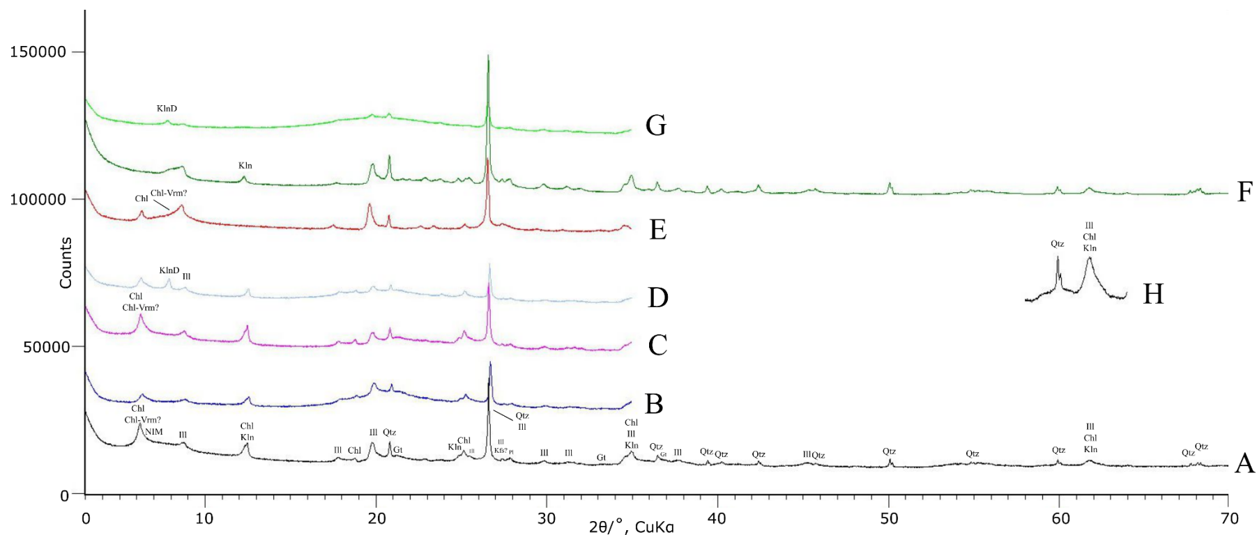
Prilog 4. Difrakcijske slike uzorka 8449 (SFL-1; 30-60 cm) frakcije < 2 \mu\text{m}
