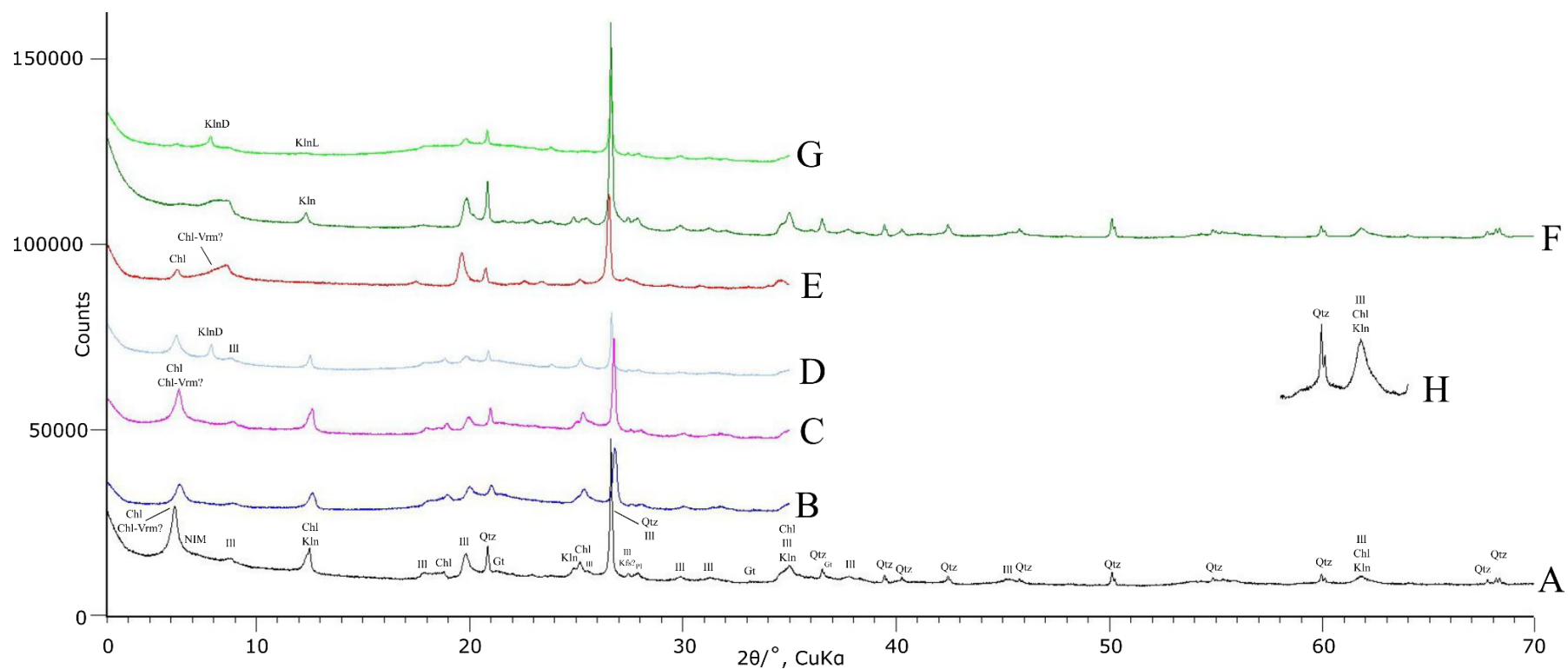
Prilog 3. Difrakcijske slike uzorka 8448 (SFL-1; 0-30 cm) frakcije < 2 \mu\text{m}
